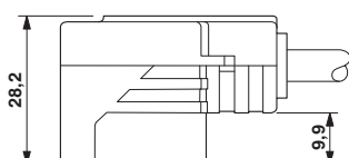
Ventilstik, type A, set fra siden
