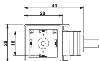
Målskitse
