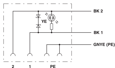
Ventilstikkets polbelægning
